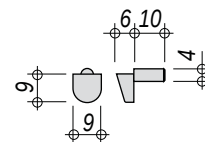
Bodenträger (bis 40kg)
